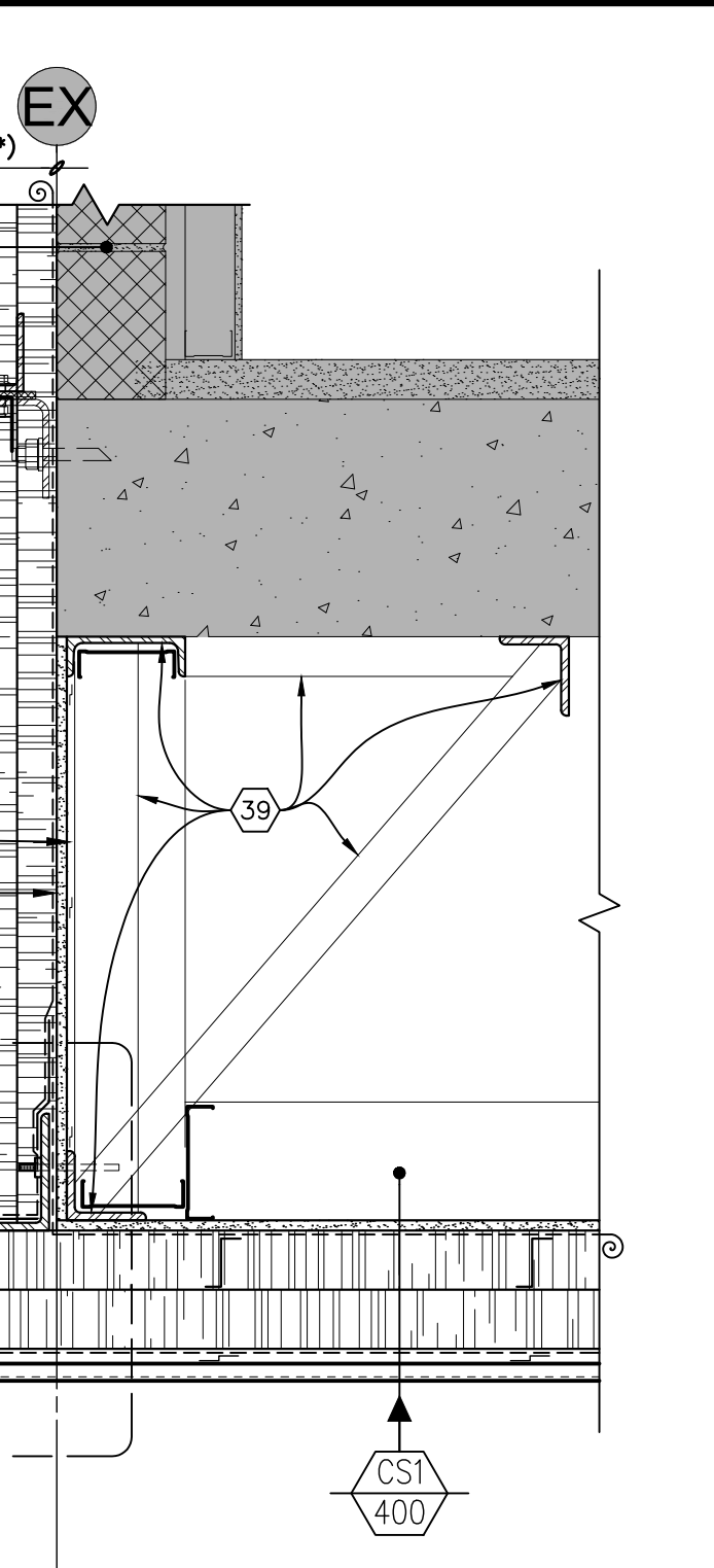
DÉMOLITION CONSTRUCTION 18 DÉTAIL TYPE PARAPET 1:10mm (GARAGE AMBULANCE)
