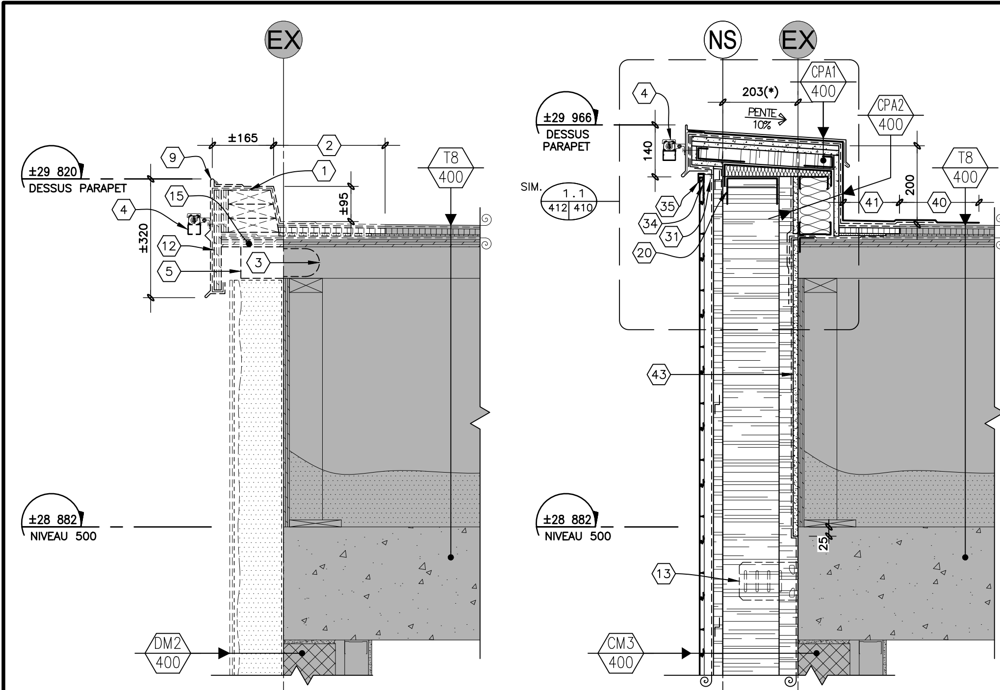
DÉMOLITION CONSTRUCTION 13 DÉTAIL TYPE PARAPET 1:10mm (TOUR ÉLEVATION OUEST)
