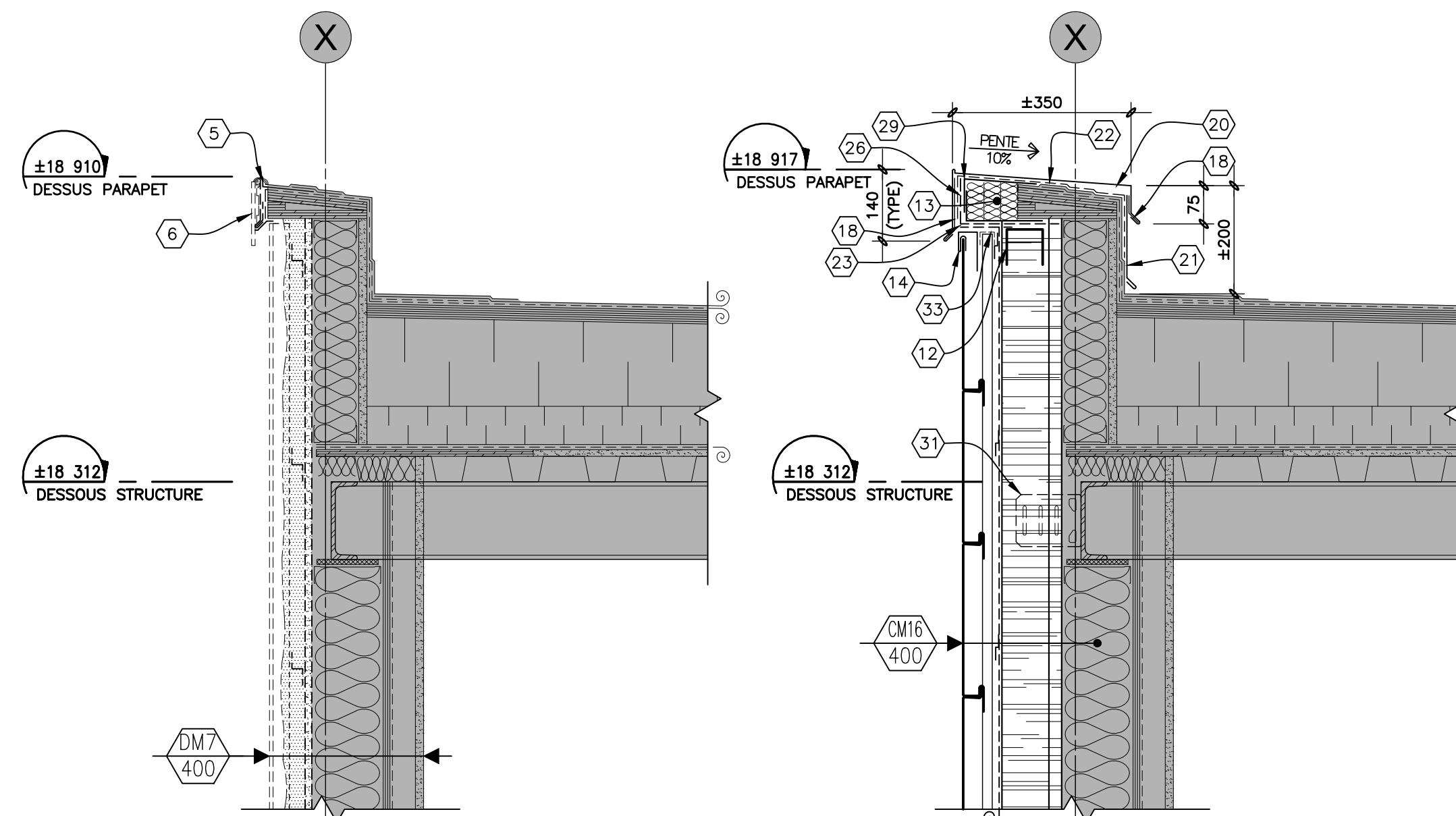
DÉMOLITION CONSTRUCTION 23 DÉTAIL TYPE PARAPET (ESCALIER #6 - ADMIN.) 1:10mm 406 413
