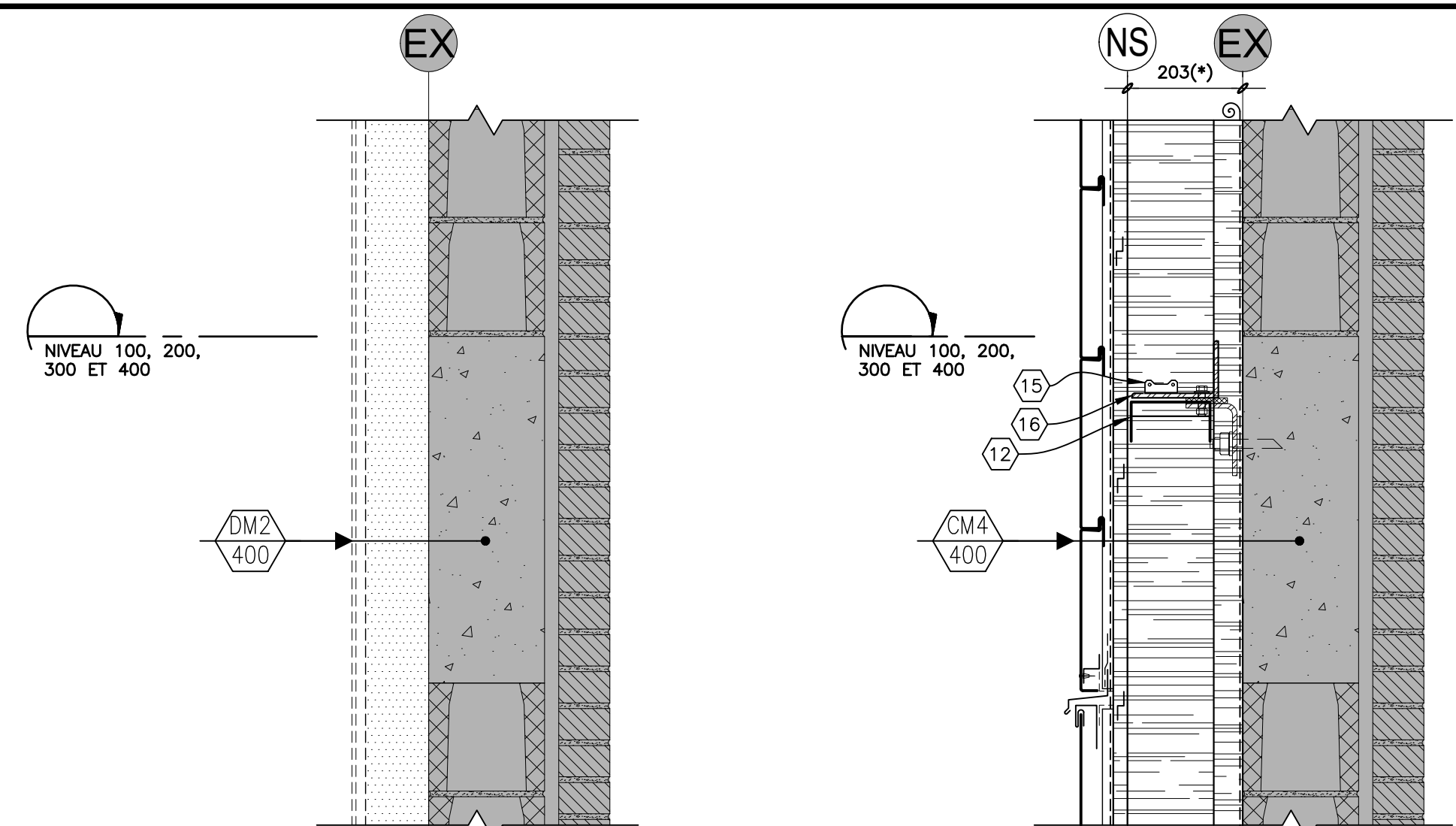
DÉMOLITION CONSTRUCTION 20 DÉTAIL TYPE (ESCALIER #3 - TOUR) 1:10mm 406 413
