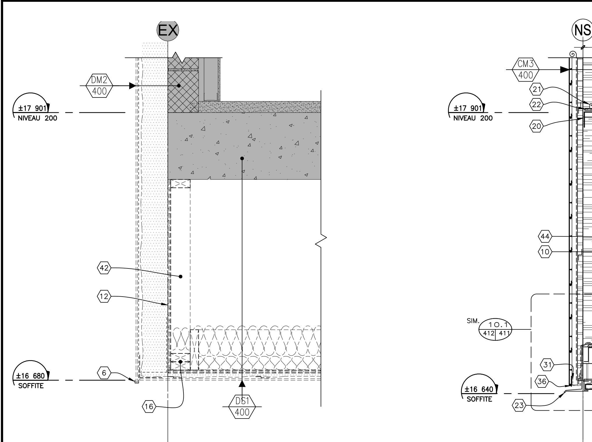
DÉMOLITION CONSTRUCTION 15 DÉTAIL TYPE PORTE-À-FAUX 1:10mm (TOUR ÉLEVATION OUEST)
