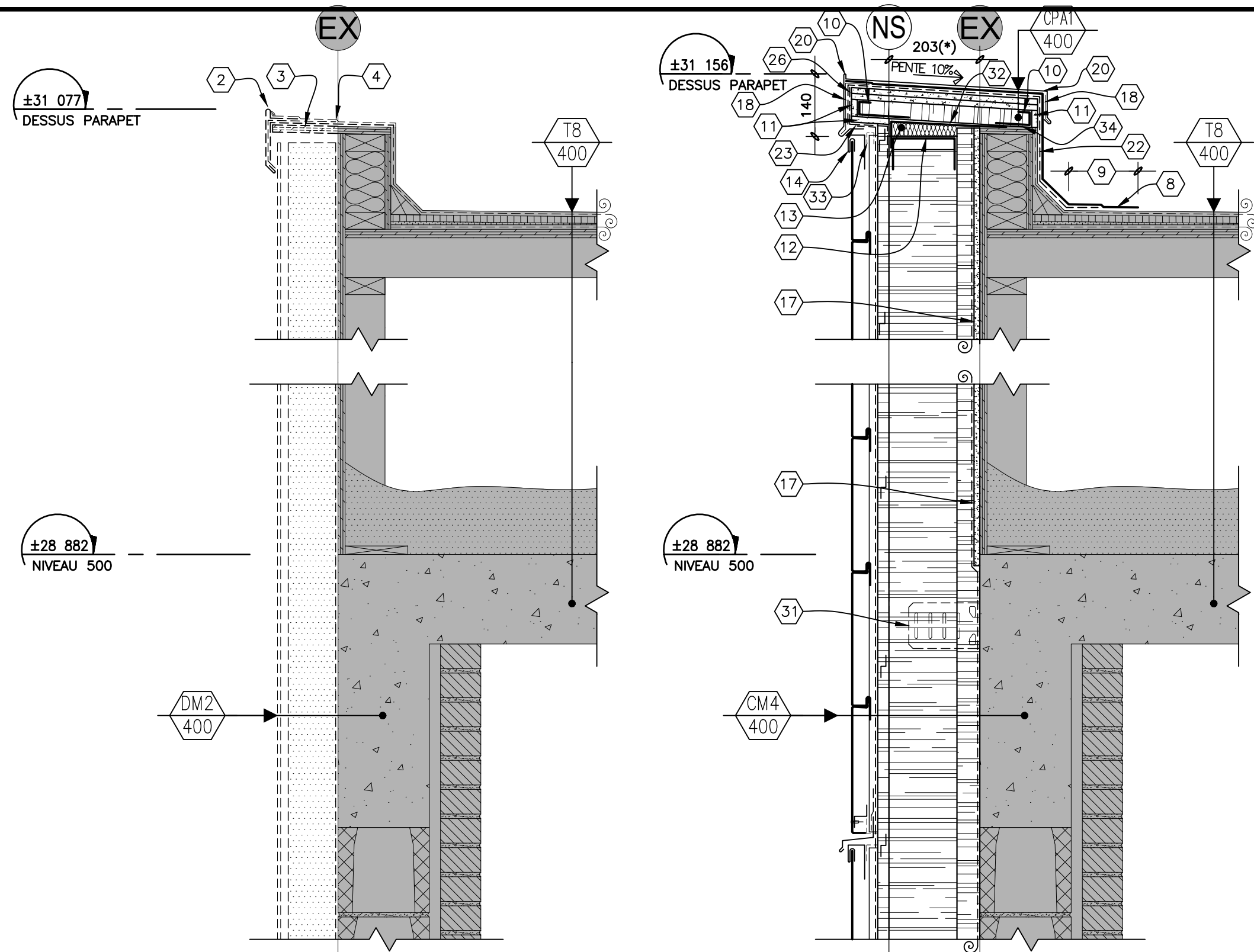
DÉMOLITION CONSTRUCTION 19 DÉTAIL TYPE PARAPET (ESCALIER #3 - TOUR) 1:10mm 406 413
