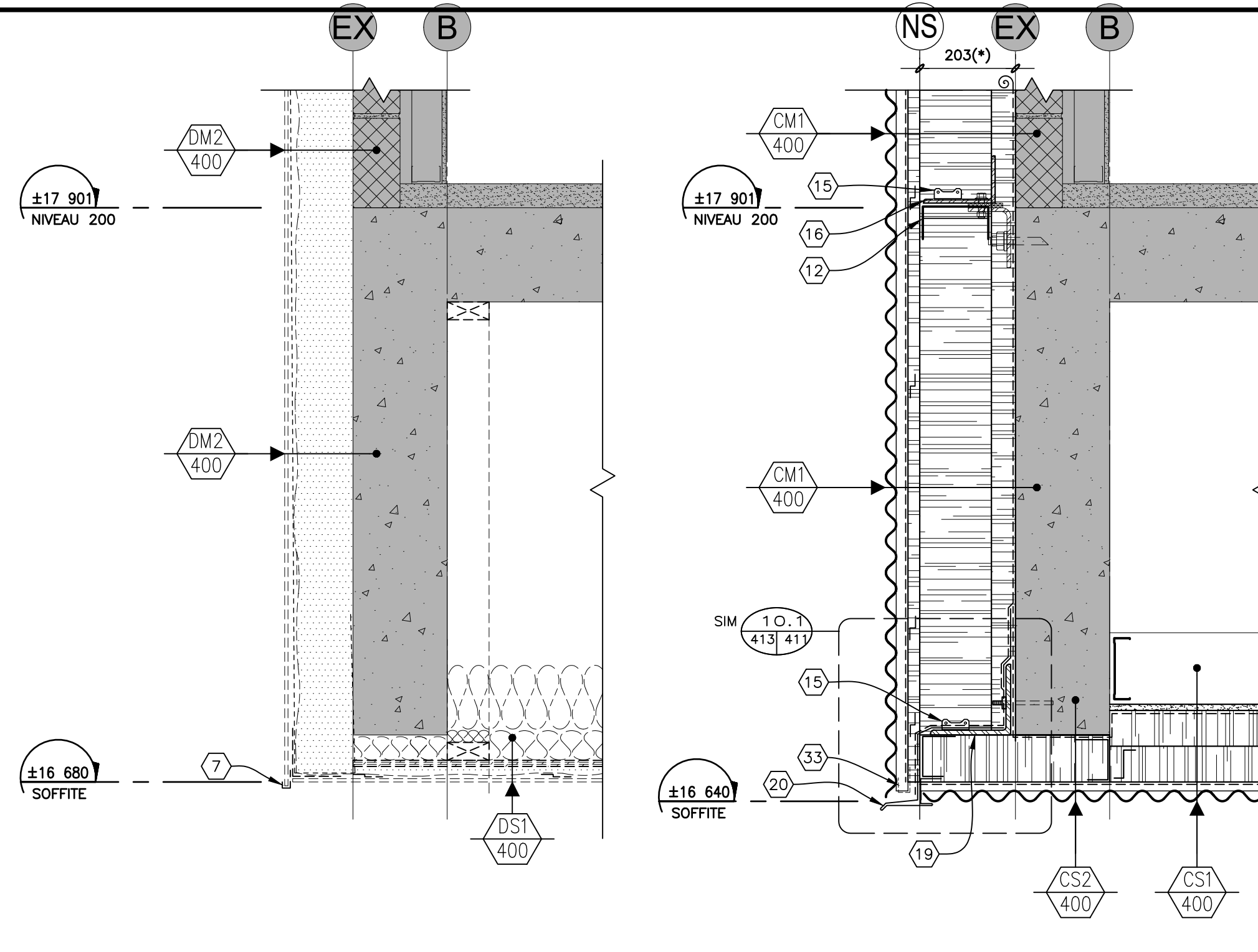
DÉMOLITION CONSTRUCTION 22 DÉTAIL TYPE PORTE-À-FAUX (TOUR/BASILAIRE NORD-EST) 1:10mm 405 413
