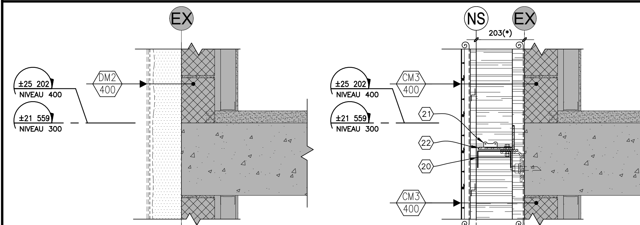
DÉMOLITION CONSTRUCTION 14 DÉTAIL TYPE 1:10mm (TOUR ÉLEVATION OUEST)
