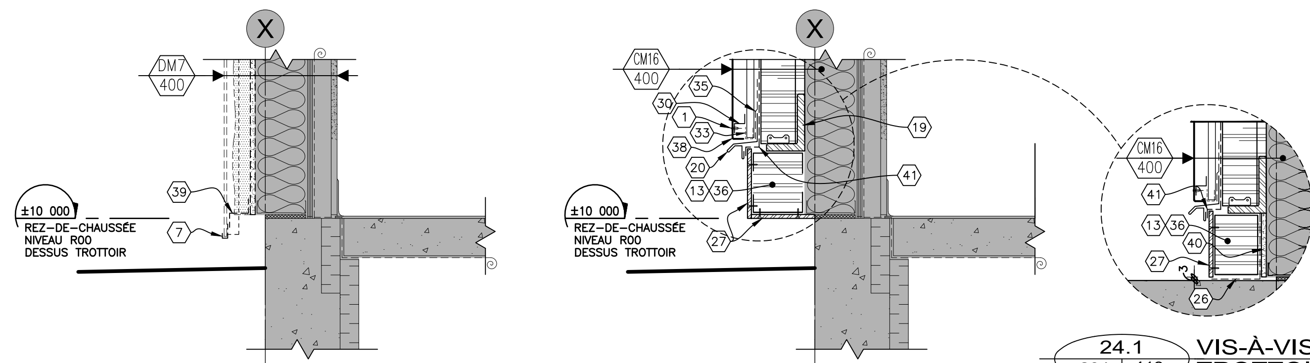
DÉMOLITION CONSTRUCTION 24 DÉTAIL TYPE (ESCALIER #6 - ADMIN.) 1:10mm 406 413
